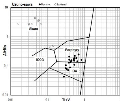
図2 磁鉄鉱の微量成分による鉱床型判別図(Nadoll et al., 2014)
